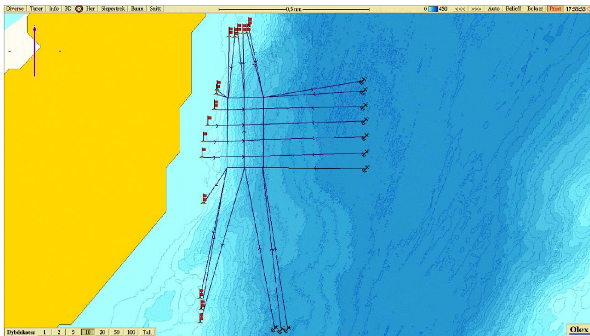
Figur 3: Oversiktskart over batymetri ved Jakobsteinsvika med dybdekoter på 10 meter. Blåtoner fra lyst til mørkt markerer økende dybde. Anleggsramme og fortøyninger er inntegnet. Kilde: Olex.
